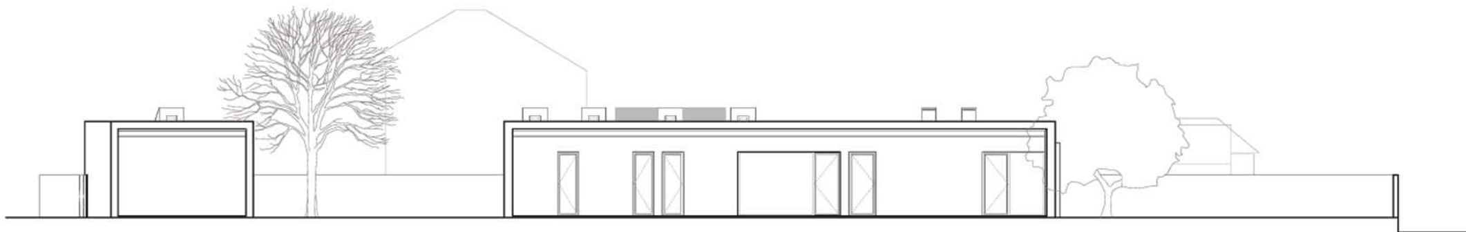
Alçado Sul - Casa do Casal do Peso
